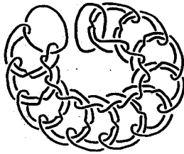
Un nœud borroméen à 13 ronds
